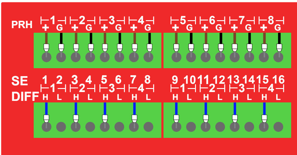
設定ファイルMIJ02LMS-08.esfを使って8本接続した例
