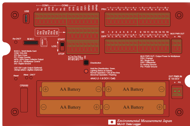
MIJ-01 Data Logger
