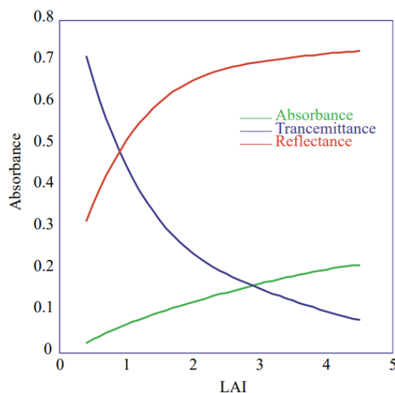
図2. LAIと吸収、透過、反射スペクトルの模式図 Absorbance;吸収
