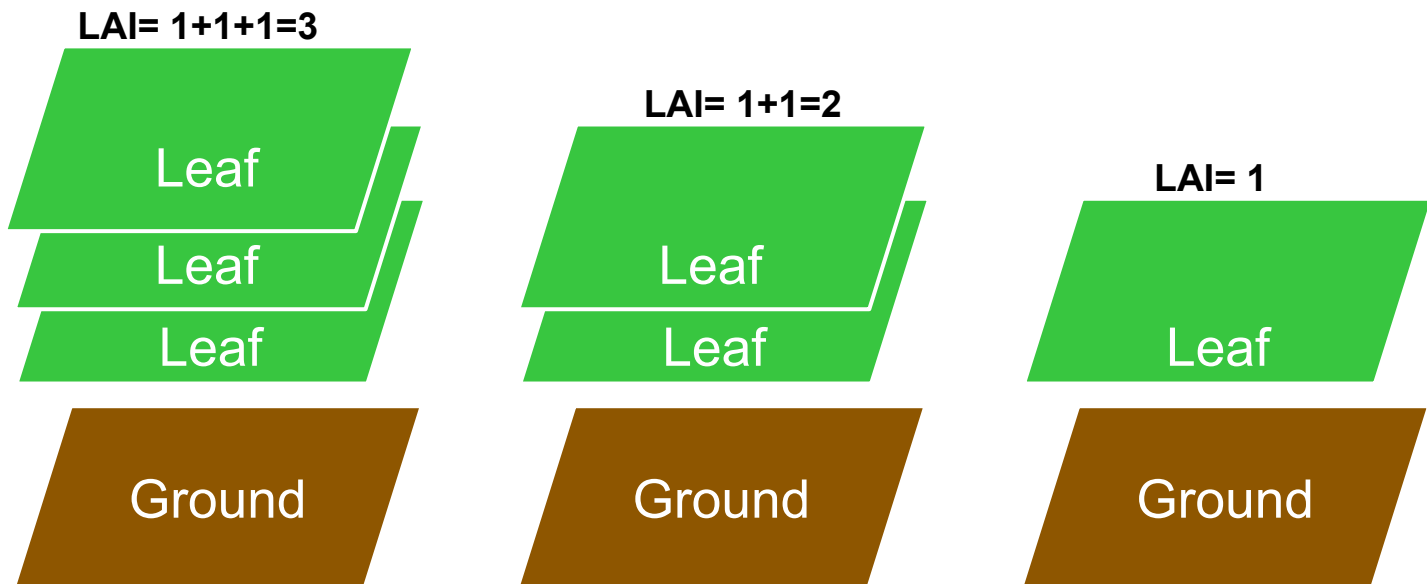
図5. LAI定義の模式図。1層に巨大な1枚の葉が存在していると仮定
