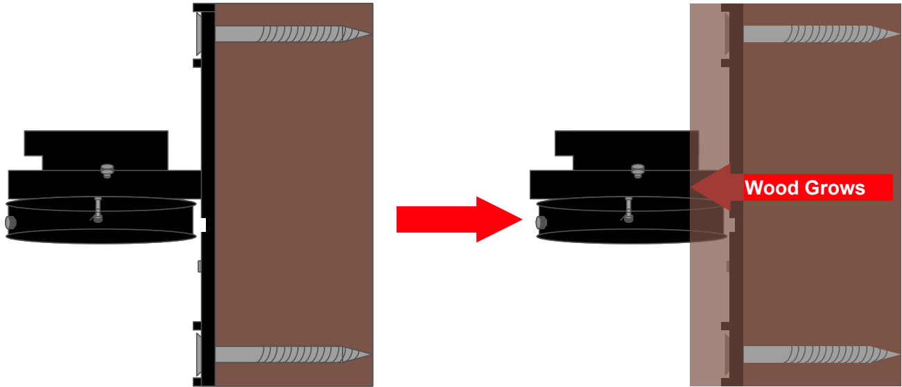
通常ねじ止め設置
