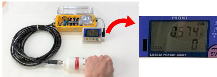
SM150Tを手で握ると図のように水分量が上がっているのが確認できます。
